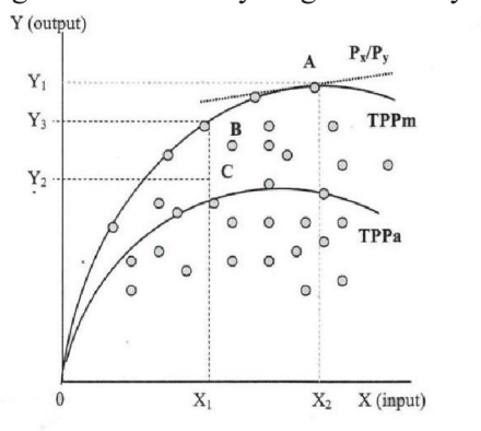
Fig 1. Frontier Production Function
