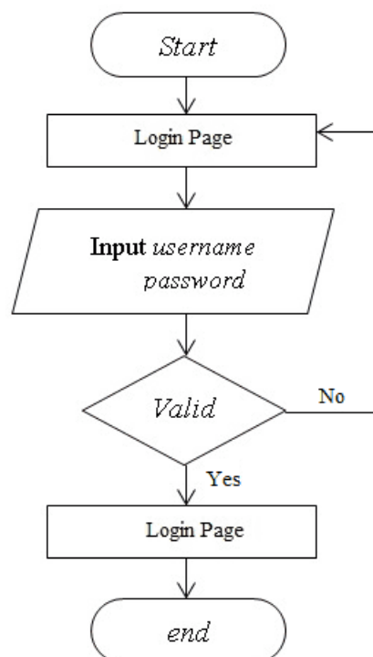
Fig 16. Flowchart login
